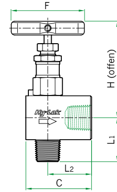
Winkelausführung
