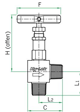
Winkelausführung
